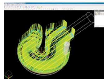
Speedy3dcomによる3次元加工
